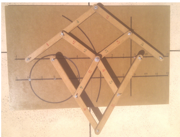
FIGURE 2 – L'additionneur est composé de deux pantographes : un en haut et un en bas. Pour la construction, les chiffres rouges indiquent la hauteur des tiges. Le chiffre 1 correspond à la barre la plus basse, elle n'est que légèrement surélevée par rapport au plateau. Sur cette photo, on calcule 2 + 9 = 11 .
