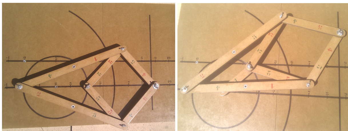
FIGURE 3 – L'inverseur de Peaucellier réalise une inversion par rapport à un cercle (photo de gauche). Les chiffres bleus indiquent la hauteur des tiges. Sur cette photo, on calcule 36/4 = 9 . En ajoutant la petite barre en bois (photo de droite), on le transforme en un mécanisme qui trace une ligne droite.
